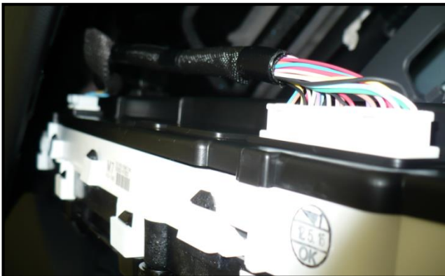
Localización del conector H62 en el cuadro
