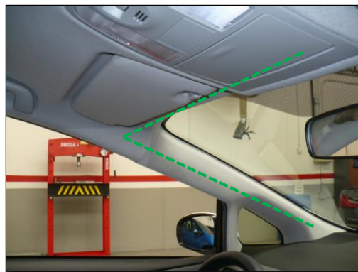
Recorrido de los cables del taxímetro de espejo
