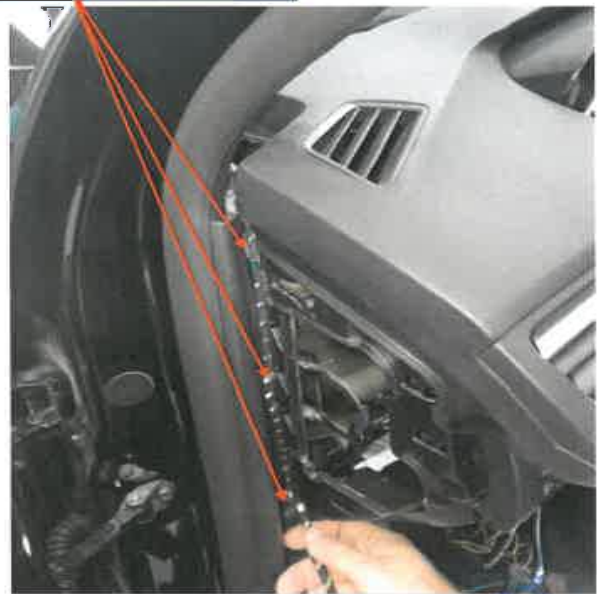
Posición mazo módulo Tarifario
