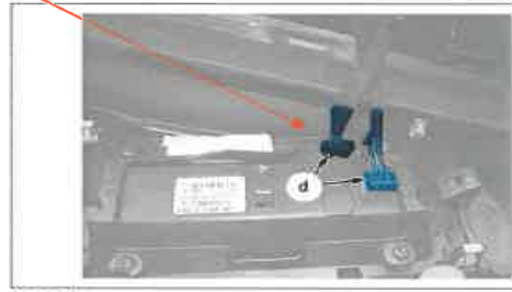
Figura CP921UD Desconectar los conectores (en "d")
