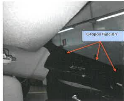
Posición mazo módulo Tarifario
