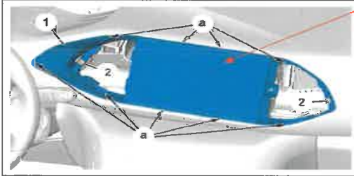
Figura CP921UD Desmontar los tornillos (2). Soltar el embellecedor (1) (en "a"). Con ayuda del úo (1350-ZZ) Soltar el embellecedor (1)
