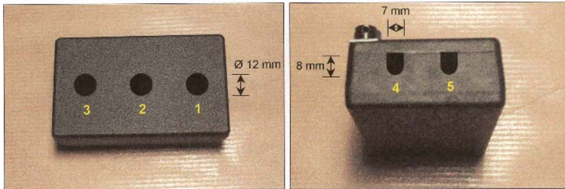
Vista inferior
