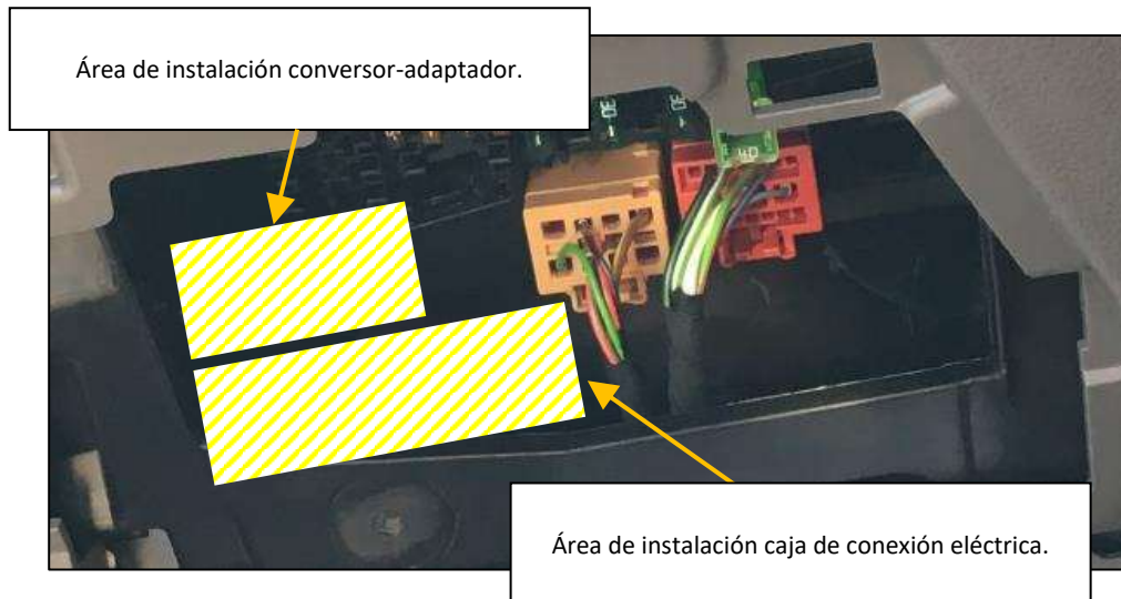
Figura 36. Área de instalación del conversor-adaptador.
