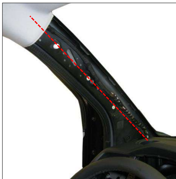
Figura 40. Recorrido del cable del taxímetro.
