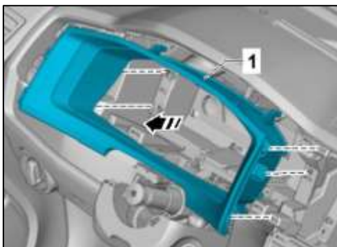
Figura 7. Desmontaje embellecedor.
