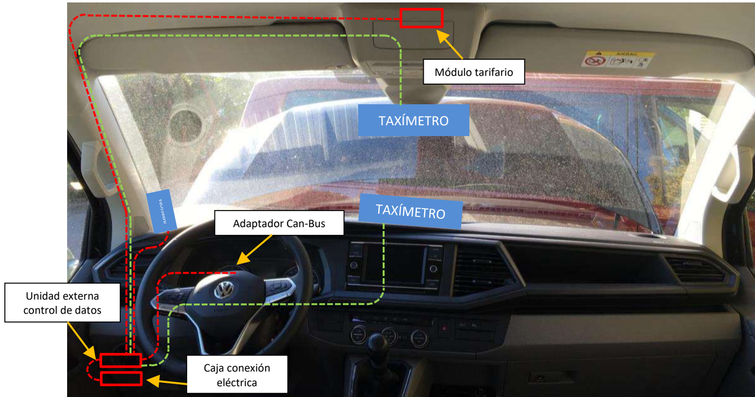
6.8. ESQUEMA DE INSTALACIÓN TAXÍMETRO CON UNIDAD EXTERNA DE CONTROL DE DATOS (TABLERO/ESPEJO) (MADRID)
