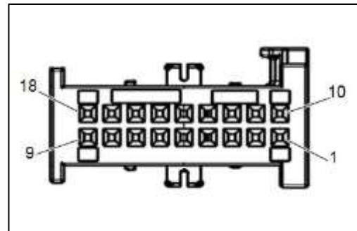
Figura 11. Detalle conexiones.
