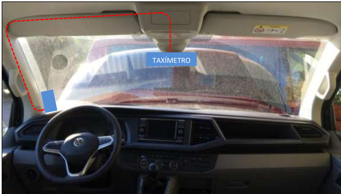
Figura 45. Recorrido cable de la impresora.
