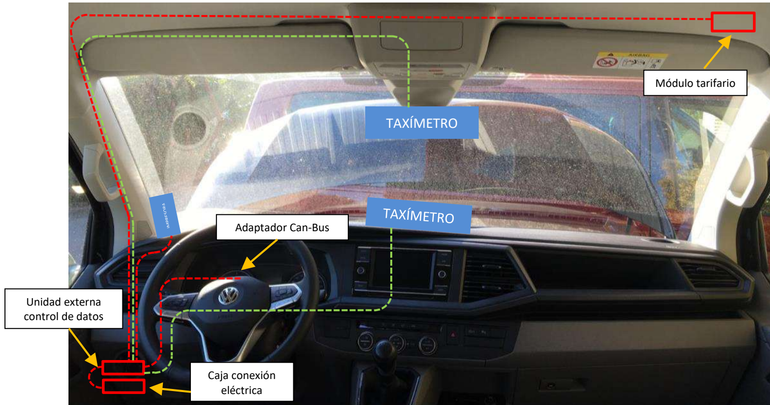
6.7. ESQUEMA DE INSTALACIÓN TAXÍMETRO CON UNIDAD EXTERNA DE CONTROL DE DATOS (TABLERO/ESPEJO) (BARCELONA)
