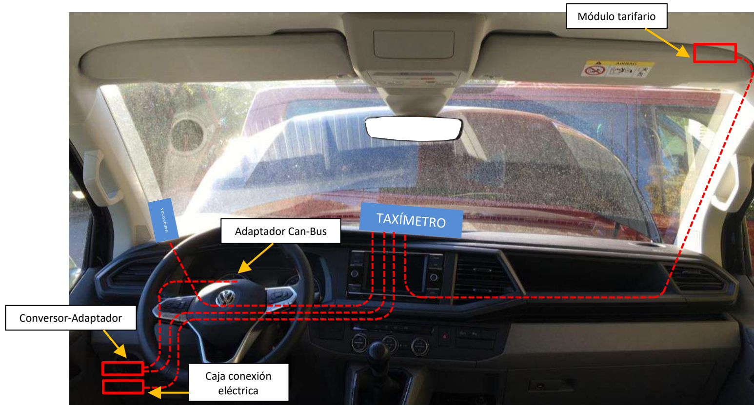
6.1. ESQUEMA DE INSTALACIÓN TAXÍMETRO CONVENCIONAL CON CONVERTOR-ADAPTADOR DE SEÑAL (BARCELONA)
