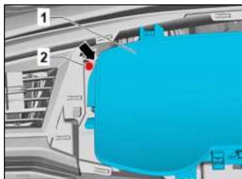
Figura 9. Detalle desmontaje cuadro de instrumentos.
