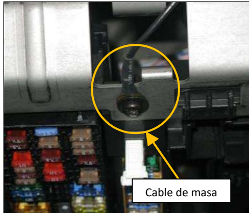
Figura 5. Cable de masa.
